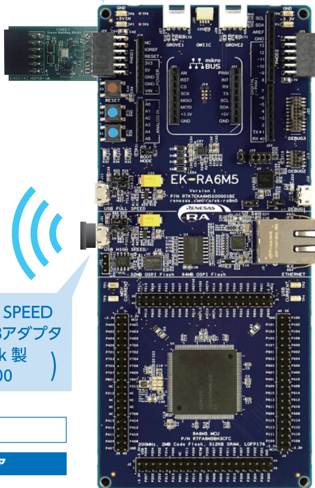
EK-RA6M5ボード
